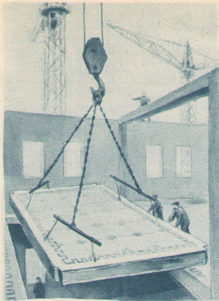
Установка крупномерной плиты межэтажного перекрытия.
