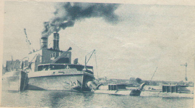
Землесос «Онега» на строительстве котлована Каховской ГЭС.
