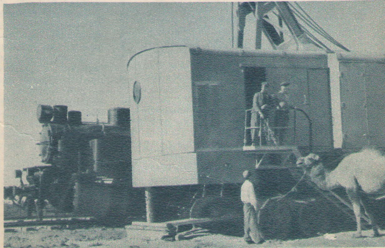
На снимке: один из трёхкубовых экскаваторов, доставленный с Уральского завода тяжёлого машиностроения. ↓
