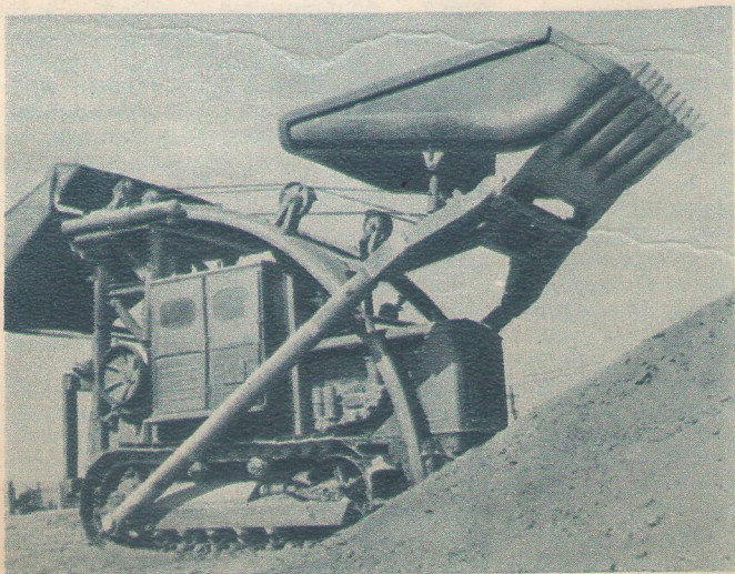
Механизированный автопогрузчик на Тахиа-Ташском участке строительства Главного Туркменского канала. ↓
